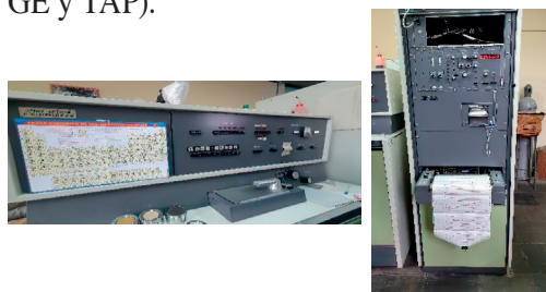
Foto 3: Equipo de laboratorio de Fluorescencia de Rayos X. (IGEMA-UMSA)
